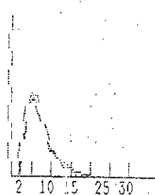
PLT HISTOGRAM
